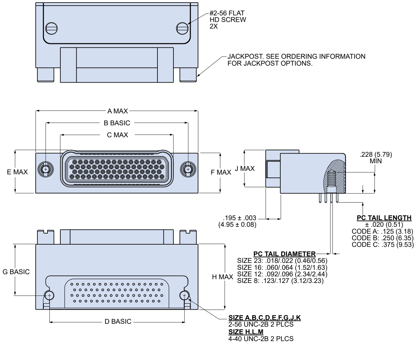
791-032P Dimensions
