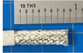
858-042-02 (0.85")
